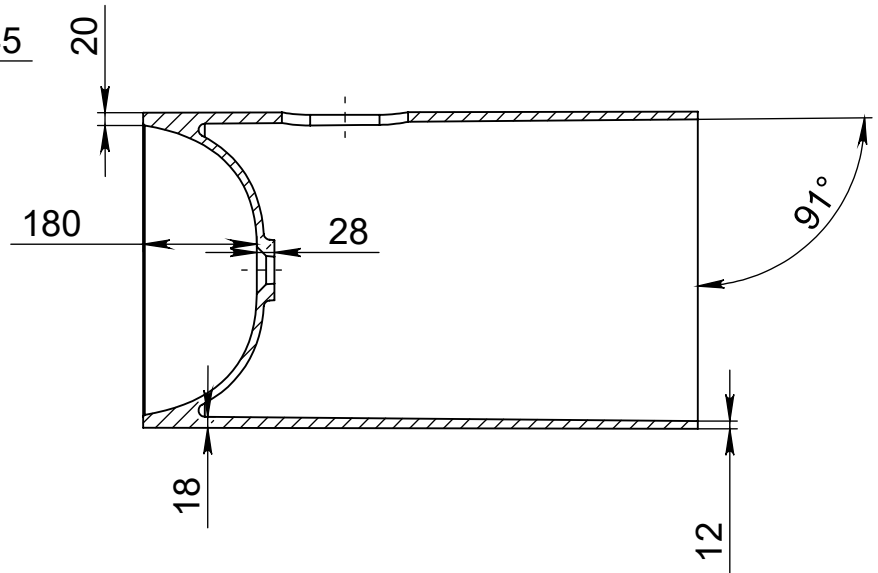
A-A
